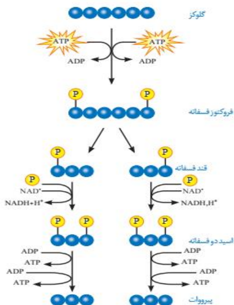
شکل ۴- مراحل قندکافت
