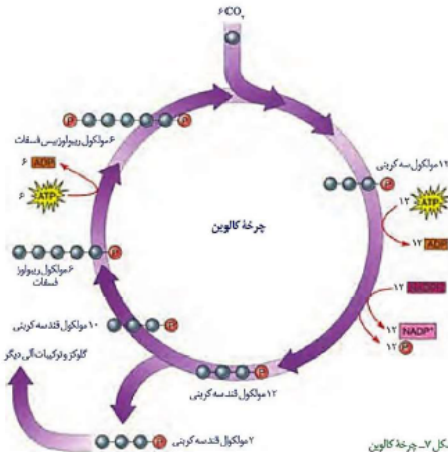
شکل ۷- چرخه کالوین
