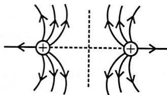
میدان الکتریکی اطراف دو بار همنام با بزرگی یکسان
