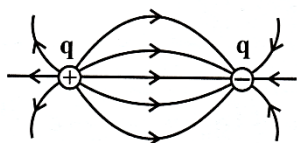
میدان الکتریکی اطراف دو بار ناهمنام با بزرگی یکسان
