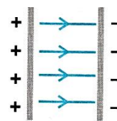
میدان الکتریکی یکنواخت بین دو صفحه رسانای باردار و موازی
