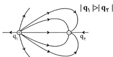
میدان الکتریکی اطراف دو بار ناهمنام با بزرگی نابرابر
