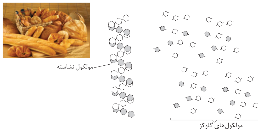
شکل ۱۹- واکنش تجزیه نشاسته و تبدیل آن به مونومرهای سازنده
