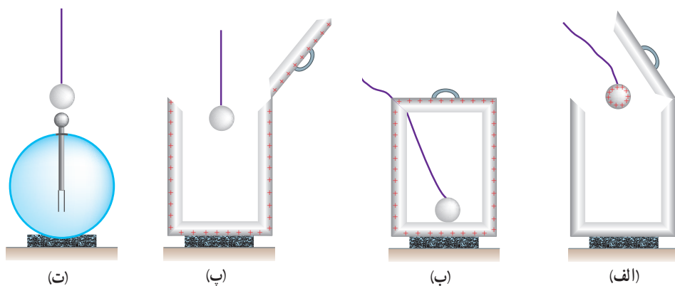
شکل ۱۷-۱ شرحی تصویری از آزمایش فارادی
