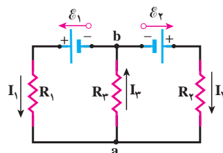
شکل ۲-۲۴ یک مدار چندحلقه‌ای که شامل سه شاخه است.
