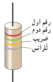
شکل ۲-۱۴ مقدار مقاومت‌های ترکیبی با کدهای رنگی مشخص می‌شود؛ مثلاً مقدار مقاومت شکل ۲۵kΩ با تولرانس ۱۰ درصد است.
