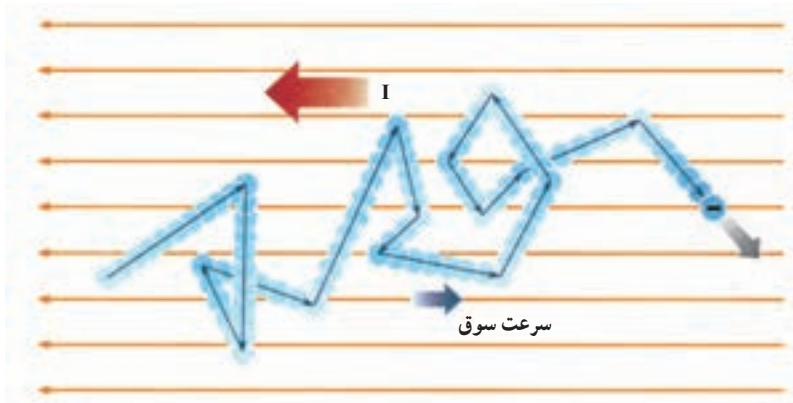
شکل ۲-۶ مسیر زیگزاگ یک الکترون آزاد در یک رسانای فلزی. در حضور میدان الکتریکی، این مسیر زیگزاگ در خلاف جهت میدان سوق می‌یابد.
