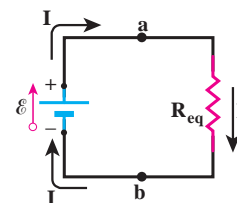
شکل ۲-۲۶ مدار معادل شکل ۲-۲۵ که در آن سه مقاومت با مقاومت معادل R_{eq} جایگزین شده است.
