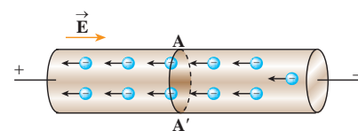
شکل ۲-۵ در حضور اختلاف پتانسیل، شارش بار خالص از مقطع AA' سیم، دیگر برابر صفر نیست.
