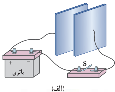
شکل ۱-۲۳ یک خازن تخت، از دو صفحه با مساحت A ساخته شده است که به فاصله d از هم قرار گرفته‌اند.
