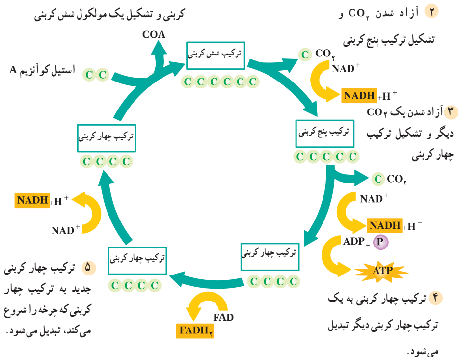
شکل ۱۲-۸ - چرخه کربس
