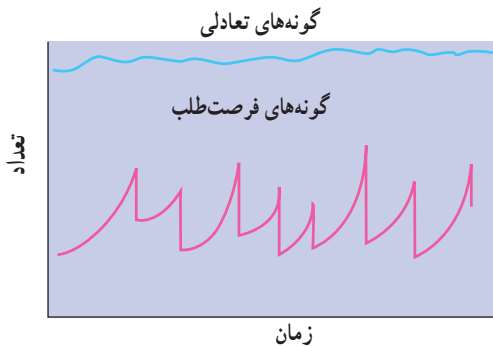
شکل ۶-۶ جمعیت‌های فرصت طلب و جمعیت‌های تعادلی
