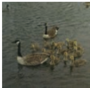
شکل ۷-۷ نقش‌پذیری در جوجه‌های غاز
