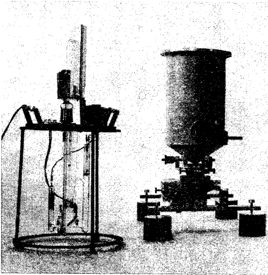
شکل ۴. یک لامپ کریپتون در آزمایشگاه‌های ملی فیزیک، تدینگتون، انگلستان. لوله شیشه‌ای در سیستم طرف چپ، حاوی گاز ^{86}\text{Kr} است. این گاز، در اثر تحریک با جریان الکتریکی، نورگسیل می‌کند. لامپ را در زمای طرف راست می‌گذارند تا آن را در دمای نیتروژن مایع ( -210^\circ\text{C} ) نگه دارد. نور از سوراخ کوچک زمای مشاهده می‌شود.
