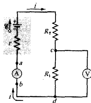
شکل ۱۴-۲۳ یک مدار تک حلقه‌ای که نشان می‌دهد آمپرسنج (A) و ولت‌سنج (V) چگونه در مدار قرار می‌گیرند.
