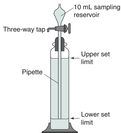
Fig. 9.12 Andreasen pipette.
