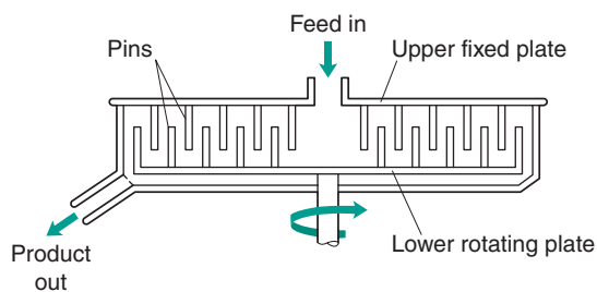
Fig. 10.14 Pin mill.
