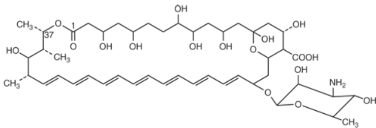
Amphotericin B
