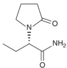
Levetiracetam
