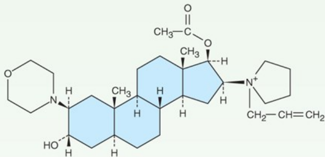
Rocuronium
