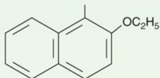
Nafcillin
