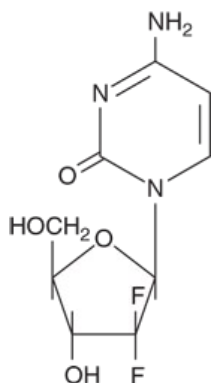
Gemcitabine
