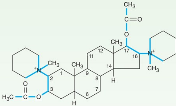
Pancuronium
