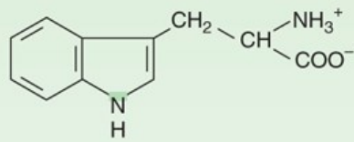
L-tryptophan
