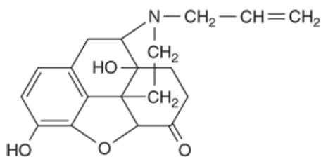
Naloxone
