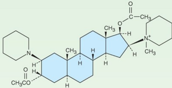
Vecuronium
