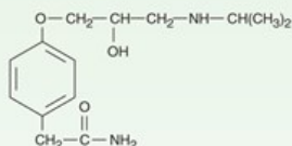
Atenolol
