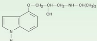
Pindolol
