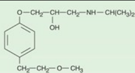
Metoprolol
