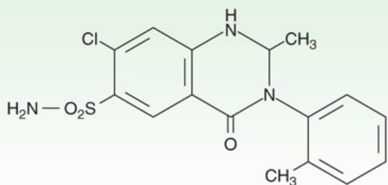
Metolazone
