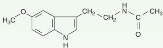
Melatonin
