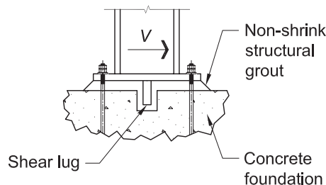
Fig. 4-25. Shear lug detail.
