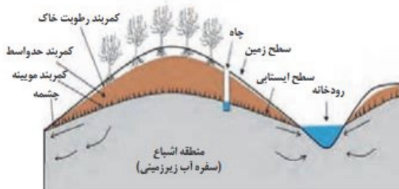
شکل ۳-۳ الف) توزیع آب زیرزمینی در خاک، ب) کمر بندهای منطقه تهیه
