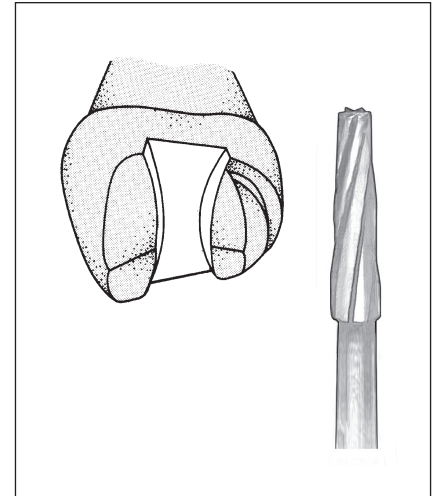
Fig 12-18 Isthmus: no. 171L bur.
